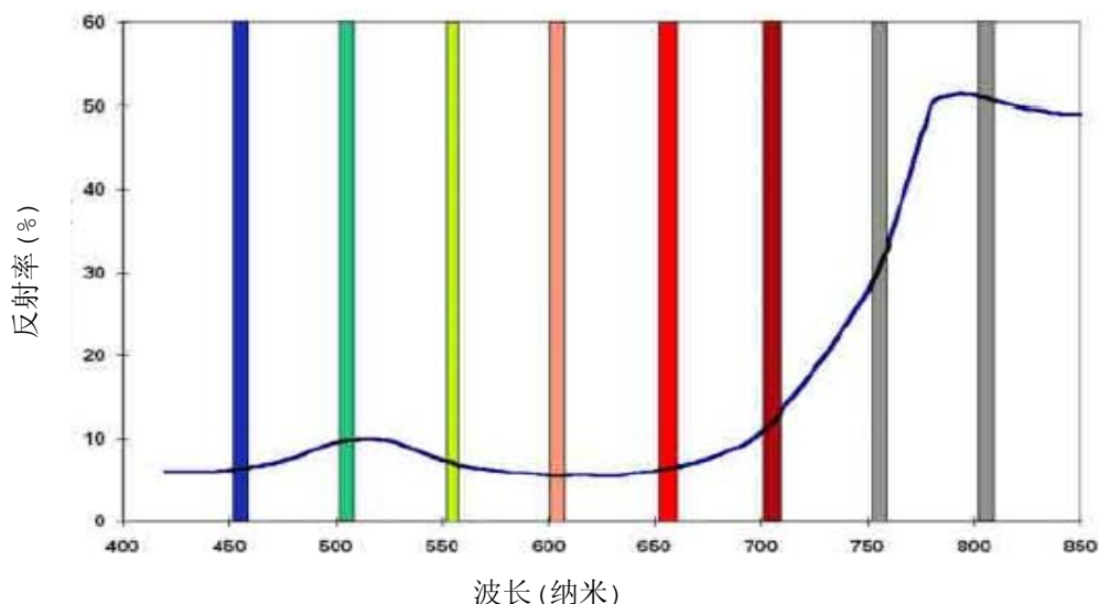
MSR5光谱波段显示典型绿色植被反射率
